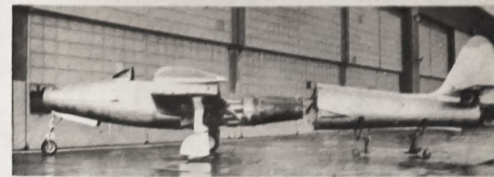
Nowy samolot amerykański «P-84 Thunderjet» jest tak skonstruowany, że można go z łatwością rozłamać na dwie połowy. Umożliwia to maksymalne wykorzystanie hangaru, co jest niezwykle ważne w czasie operacji, jak to wykazuje doświadczenie z ostatniej wojny. Samolot wyposażony jest w napęd rakietowy i przypuszcza się, że jego szybkość będzie nie mniejsza niż 600 mil na godzinę, chociaż wszystkie bliższe szczegóły dotyczące nowego samolotu trzymane są w ścisłej tajemnicy
