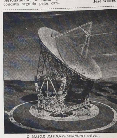
Em desenho, vê-se o maior rádio-telescópio móvel do mundo, construído nos Estados Unidos perto de Sugar Grove, na Virgínia Ocidental. Sua construção custou 79 milhões de dólares e permitiu que se sintonizassem sinais radiofônicos de corpos celestiais que se encontram a 38 bilhões de anos-luz, ou seja, 19 vezes mais do que a distância percorrida pelo telescópio de Monte Palomar. O instrumento pesa 20 mil toneladas e tem um prato refletor de 180 metros de diâmetro. A altura do rádio-telescópio é equivalente a de um edifício de 55 andares.
