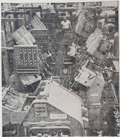
AUTOMATIZAÇÃO Numa fábrica de Detroit, esta gigantesca máquina fabrica automaticamente peças para motores de automóveis. A automatização aumentou a necessidade de operários altamente especializados em máquinas norte-americanas. No adiantamento de 140 trabalhadores substituídos por máquinas, que possam desempenhar outras tarefas, colaboram os sindicatos, as firmas industriais e entidades do governo.
