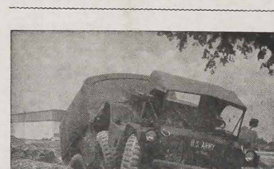
W Stanach Zjednoczonych wyprodukowano nowy samolód ciężarowy, którego przyczepka przybiera pozycję stosownie do nierówności terenu. "Kaminion" ten można przewozić na helikopterach i zrzucać go przy pomocy specjalnego spadocznika.
