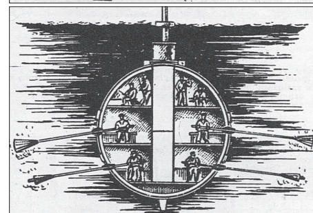
Okręt podwodny Czarnowskiego wg rysunków z Państwowego Muzeum Białorusi w Mińsku
