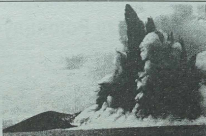
Wulkan-junior. Nawet po wielkim wybuchu z 1883 roku Krakatau nie uspokoił się. W roku 1928 z morskich odłamków wyłania się Anak Krakatau - dziecko Krakatau. W ciągu następnych lat wysępka ta zapadała się trzykrotnie, by pojawić się ponownie jeszcze cztery razy.
