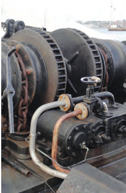
Паропровод к судовой лебёдке
