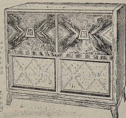
PHILCO TROPIC 3113 - Ondas curtas e longas com 5 faixas ampliadas para sintonização. 7 Válvulas. Ligação para toca-discos. Alto falante de 7 polegadas. Caixa de desenho moderno em madeira escura.
