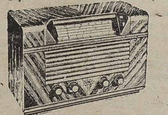
PHILCO TROPIC 3514 - Ondas curtas e longas. 5 faixas de sintonização. 6 possantes válvulas. Ligação para toca-discos. Bela e sobria caixa de madeira esmerilhada. Funciona com corrente elétrica de 110, 220 volts ou acumulador de 6 volts.
