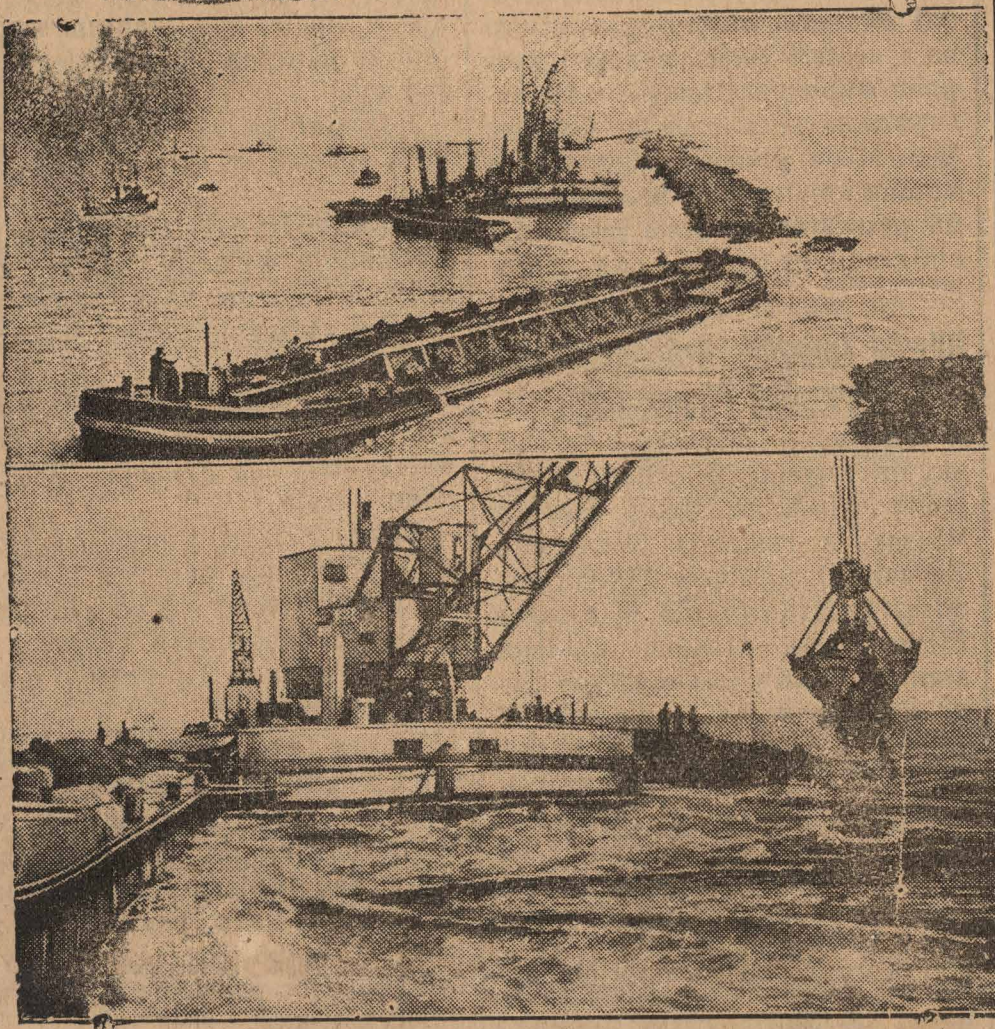
1) Port w budowie. 2) Dźwigar portowy przy pracy.
