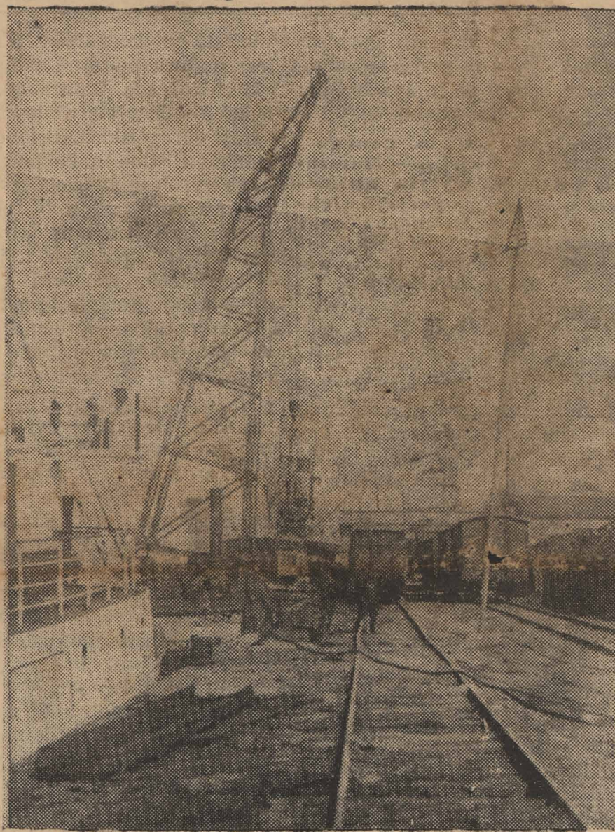
Ustawianie dźwigów skarbowych firmy M. A. N. na nabrzeżu Polskiem basenu im. Marszałka Józefa Piłsudskiego.
