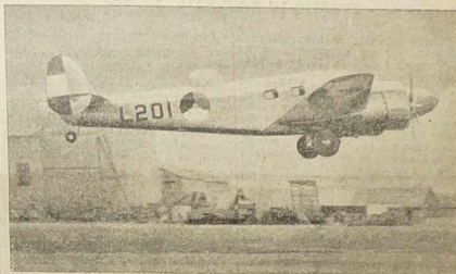
Najnowy model amerykańskiego samolotu bojowego Lockheed 212, który rozwija szybkość 400 km. na godz. — Holandia zakupiła 12 takich samolotów dla Indji Holenderskich.
