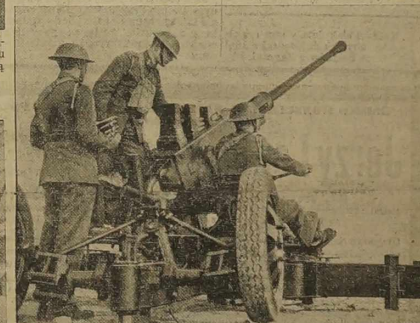
Angielskie szybkostrzelne działko przeciwlotnicze w chwili zajęcia pozycji gotowej do ostrzeliwania samolotów nieprzyjacielskich.
