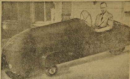
Ten niezwykły samochód zbudował sobie handlarz farb, J. Grady Tingle z Miami, na Florydzie. Boczne małe kółka utrzymują jedynie auto w równowadze, gdy stoi. W czasie jazdy samochód używa tylko 2-eh kół.
