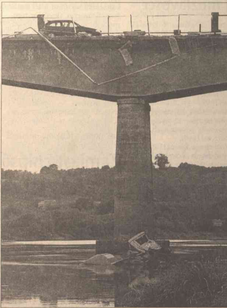
W poniedziałek pod wieczór z mostu do rzeki Nevėžis (rejon kowieński), po złamaniu ogrodzenia, wpadła betoniarka, należąca do spółki „Vilijampolės gelžbetonis”. Kierowca większych obrażeń nie doznał. Okoliczności wypadku bada się. Fot. ELTA
