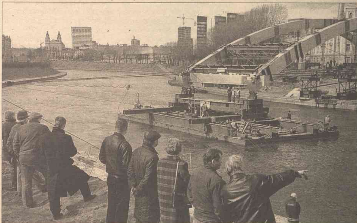
W celu odholowania ogromnej metalowej konstrukcji mostu na przeciwny brzeg został wykorzystany zbudowany z 16 pontonów prom, działający na zasadzie statku podwodnego Fot. Marian Paluszkiewicz
