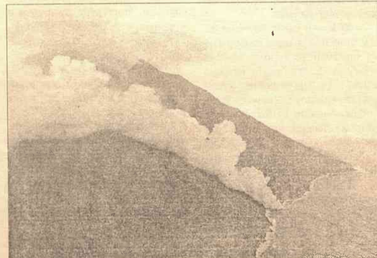
Na wyspie Stromboli rozszarżona do białości lawa splywa po zboczach wulkanu, nad którym się unosi słup pary wodnej. Zdjęcie wykonane zostało w czwartek, 2 stycznia.
