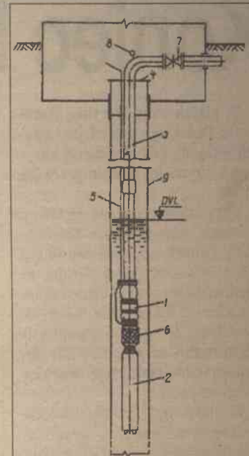
Pompa głębinowa z silnikiem zatopionym
