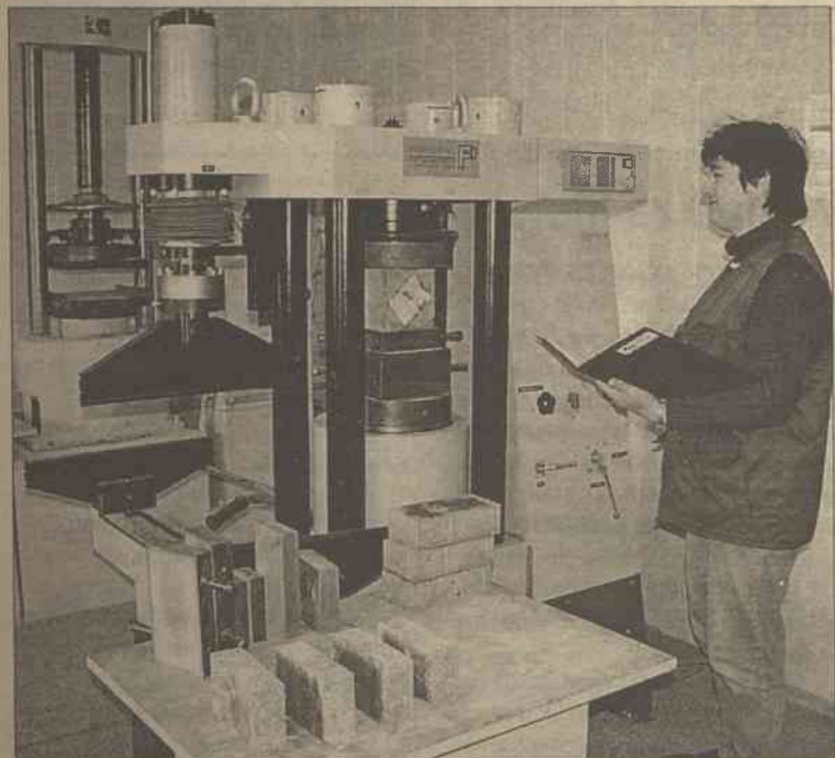
Beton również wymaga bardzo precyzyjnych badań laboratoryjnych — mówi laborantka Tajana Michniewicz
