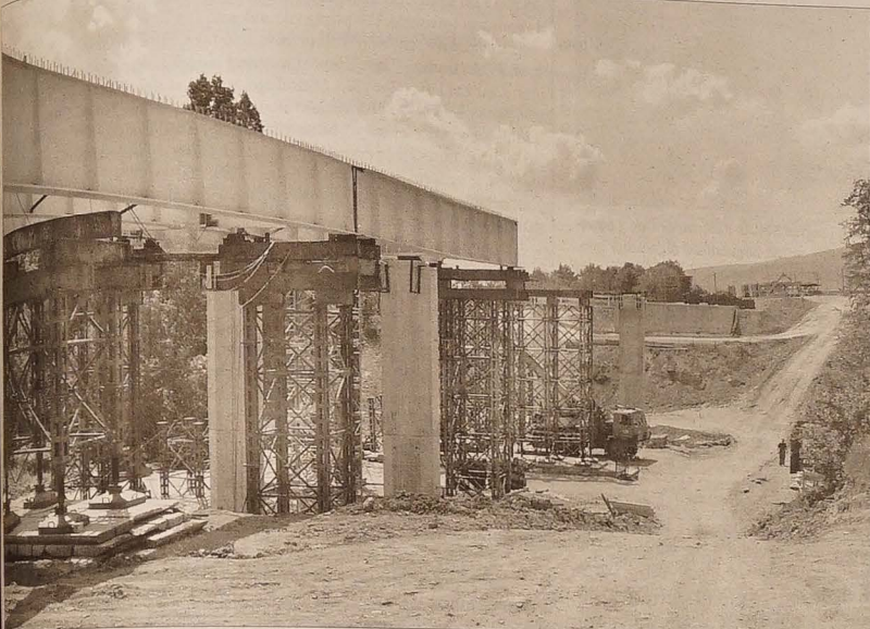
Most, po którym już w sierpniu powędzie ruch kołowy nad Jasynińskim Potokiem na budowanej obwodnicy Jablonkova 1/11 został przeznaczonej na plac budowy, gdzie czekają prace montażowe i betoniarskie. Most wykonały Zakłady Maszynowe w Trzyńcu – siedziba firmy Hutny Trzinec.
